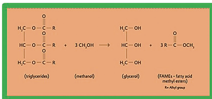
Figura 1. Reacción para la producción de biodiésel.
