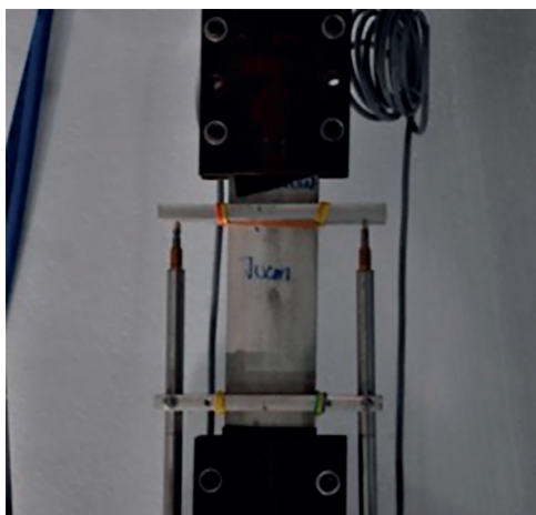
Figura 2. Ensayo de tracción directa compuesto.
